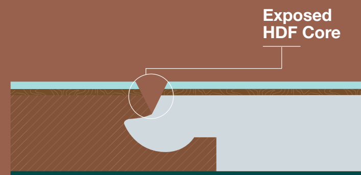
V-GROOVE (FIG.3)
