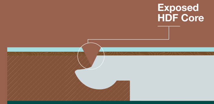
V-GROOVE (FIG.3)
